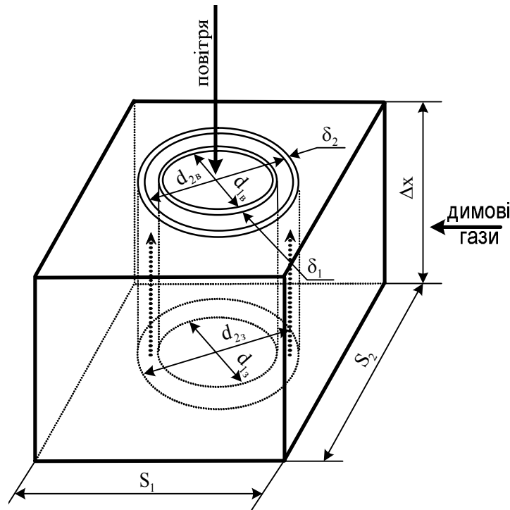
Рис. 3. Розрахунковий елемент рекуператора подвійної циркуляції
