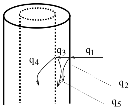
Рис. 2. Схема теплообміну в рекуператорі подвійної циркуляції
