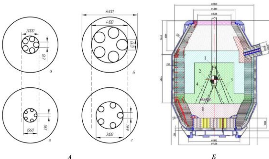
Рис. 2. А) Схема та параметри області контакту кисневих струменів з поверхнею конвертерної ванни для 5-ти соплового штатного ( \alpha = 17^{\pm 30} град) (а, б) та дослідного ( \alpha = 15^{\pm 30} град) (в, г) наконечника при висоті фурми над рівнем ванни 1,8 і 4 м відповідно; Б) Схематичне зображення розташування умовних зовнішніх границь зон контакту кисневих струменів з поверхнею ванни при різній висоті фурми, оснащеної 5-ти сопловими наконечниками: 1, 2 — висота фурми над рівнем ванни 4 і 1,8 м відповідно; 3, 4 — зовнішні границі кисневих струменів для штатного й дослідного наконечника
