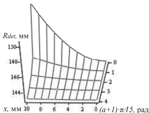
Рисунок 5 – Зміна радіуса симетричної частини деталі R_{det} за її довжиною x при умовно нульовому діаметрі шліфувального круга
